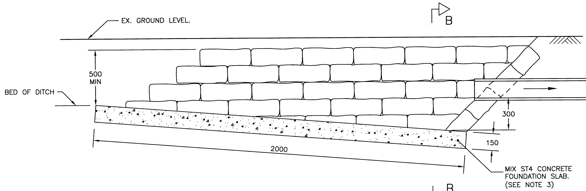
LONGITUDINAL PROFILE
