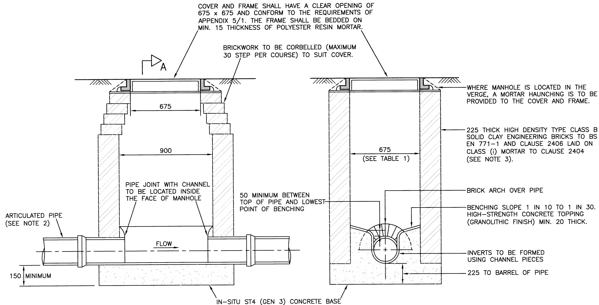
SECTION A-A
